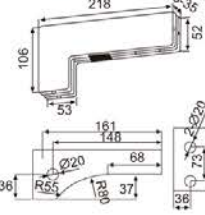
外观尺寸 Dimensions
