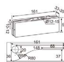
外观尺寸 Dimensions
