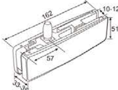
外观尺寸 Dimensions
