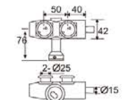
EJ-661 曲型固定件 Side panelover panel connector 主要材质: 不锈钢 Material: Stainless steel
