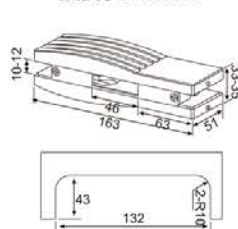
外观尺寸 Dimensions
