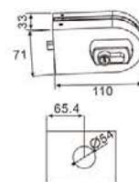
外观尺寸 Dimensions
