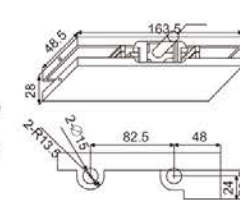
外观尺寸 Dimensions
