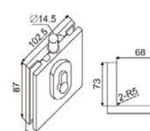
外观尺寸 Dimensions
