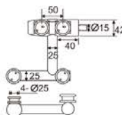
EJ-659 曲型顶轴 Side panelover panel pivot 主要材质: 不锈钢 Material: Stainless steel
