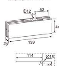
外观尺寸 Dimensions
