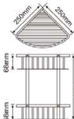
EJ-5033 置物篮 Pendant 主要材质：不锈钢 表面处理：拉丝 Material: Stainless steel Finish: Satin
