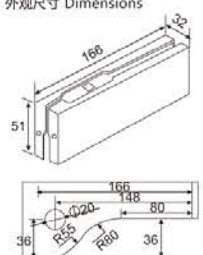
外观尺寸 Dimensions
