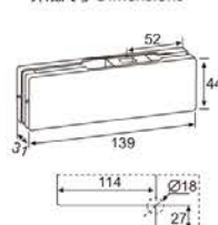
外观尺寸 Dimensions
