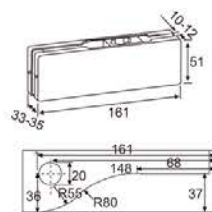
外观尺寸 Dimensions
