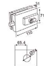
外观尺寸 Dimensions
