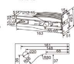
外观尺寸 Dimensions
