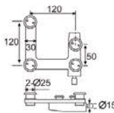
EJ-659 曲型顶轴 Side panelover panel pivot 主要材质: 不锈钢 Material: Stainless steel
