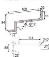
外观尺寸 Dimensions
