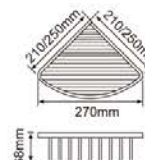
EJ-5031 置物篮 Pendant 主要材质：不锈钢 表面处理：拉丝 Material: Stainless steel Finish: Satin
