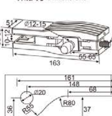
外观尺寸 Dimensions
