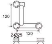
EJ-661 曲型固定件 Side panelover panel connector 主要材质: 不锈钢 Material: Stainless steel
