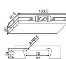
外观尺寸 Dimensions
