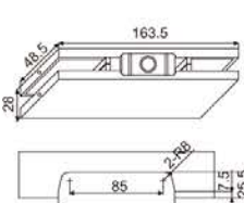
外观尺寸 Dimensions
