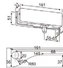
外观尺寸 Dimensions
