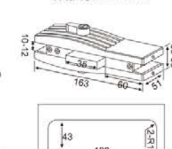
外观尺寸 Dimensions
